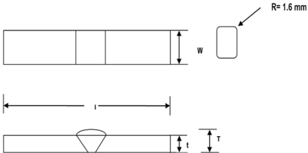
Figura 17 - Probeta de doblado guiado
